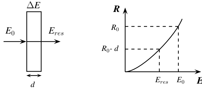
Fig. 7.4 – Principe du calcul des pertes d'énergie.
