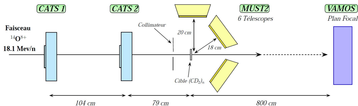
Fig. 6.2 – Schéma de principe du dispositif expérimental.
