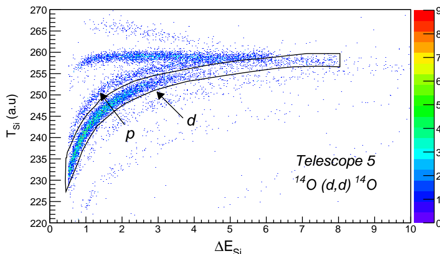
Fig. 7.8 – Identification des particules dans une matrice énergie-temps de vol donné par le silicium à piste du télescope 5 lors d'un run de diffusion élastique 14 O(d,d).
