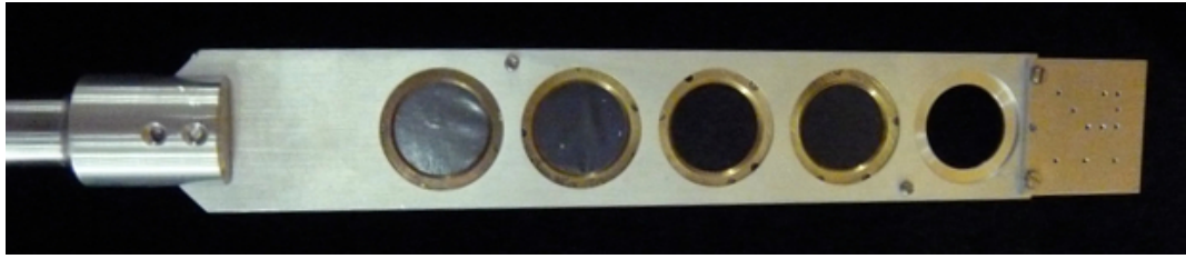
Fig. 6.5 – Image du porte cible placé verticalement dans la chambre à réaction.
